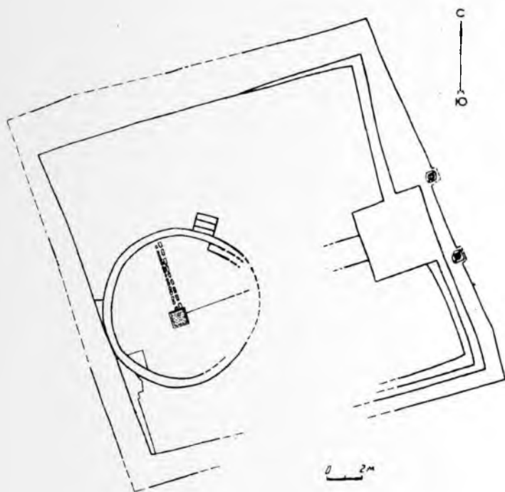
Рис. 7. Уйбатский город. План храма Миропорядка (840—841 гг.).
