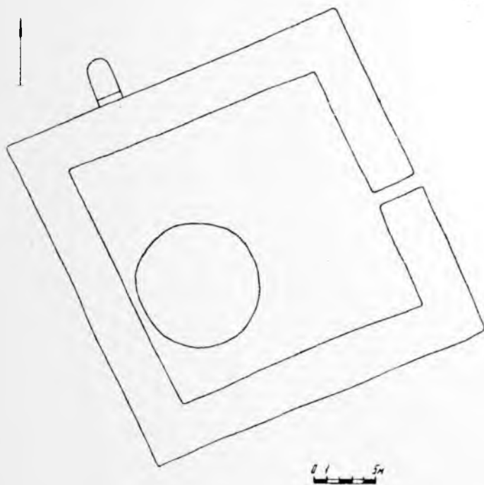
Рис. 3. Уйбатский город. План храма Первопричины (758—759 гг.) Внутри — вихар с куполом, снаружи — скругленная платформа храма Огня.
